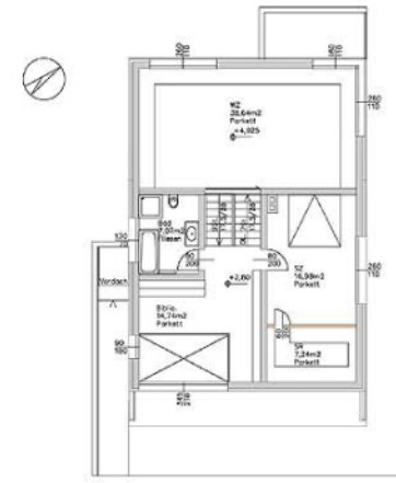
OBERSGESCHOSS +2,80 / +4,20
