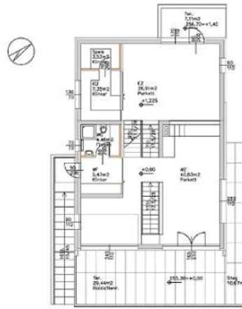
ERDGESCHOSS +0,00=255,70 / +1,40
