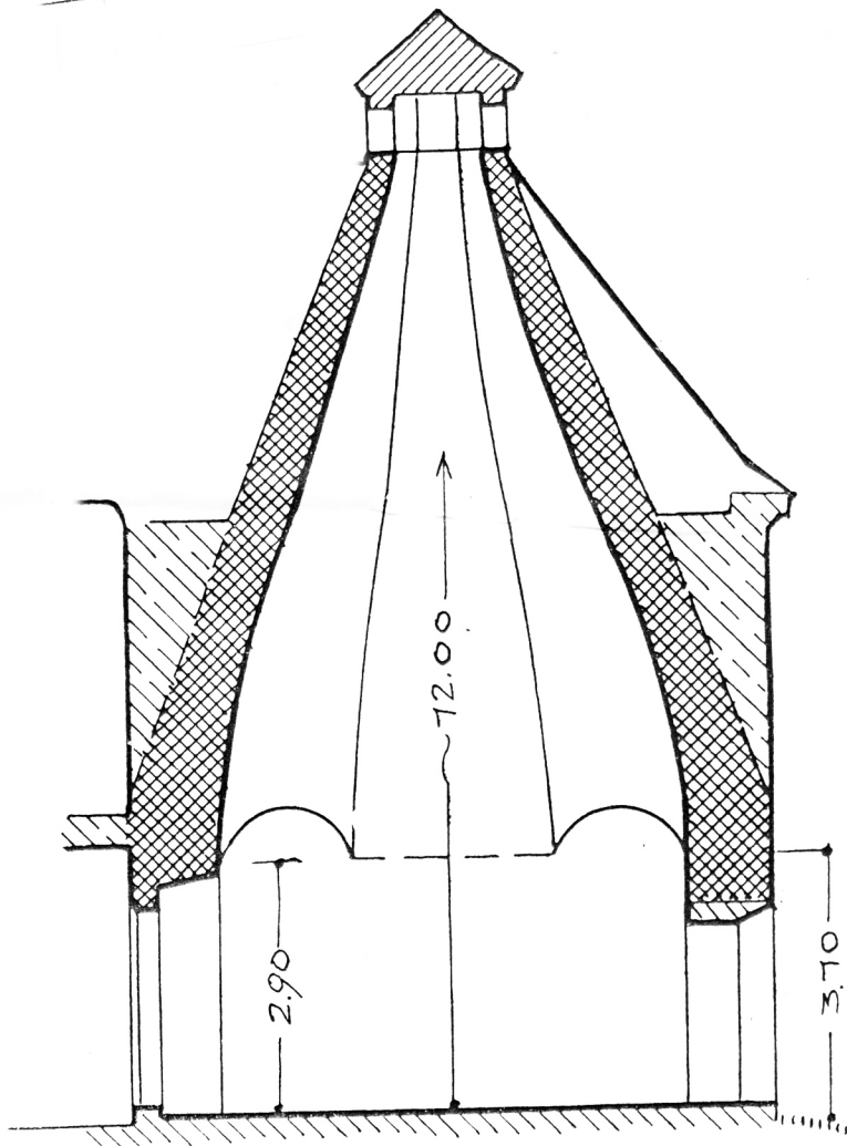
Schnitt durch die Rauchküche
